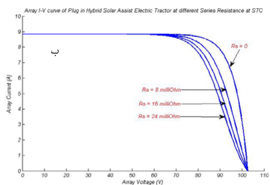
شکل ۶- تاثیر مقادیر مختلف n (الف) و افزایش R_s در کاهش سطح زیر منحنی نمودار I-V (ب)
