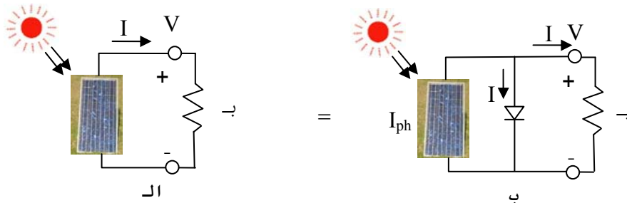
شکل ۲- مدار یک سلول خورشیدی متصل به بار (الف) و مدار هم ارز آن (ب)
