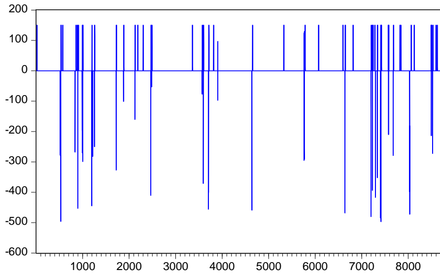
نمودار ۱- تولید لحظه‌ای-ساعتی توربین در سیستم ذخیره‌ساز هوای فشرده با ظرفیت ۱۵۰ مگاواتی
