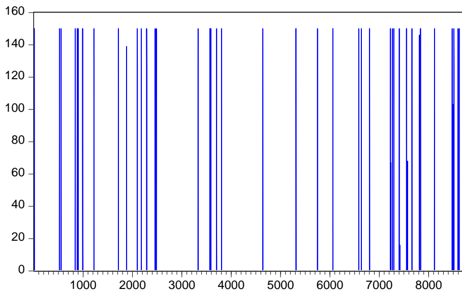
نمودار ۲- مصرف لحظه‌ای-ساعتی کمپرسور در سیستم ذخیره‌ساز هوای فشرده با ظرفیت ۱۵۰ مگاواتی
