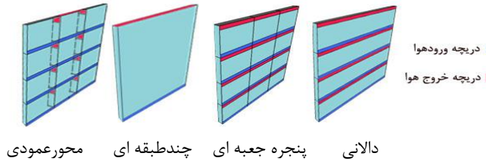
شکل ۵- دریچه های ورود و خروج هوادرگونه های مختلف نمای دوپوسته در تابستان
