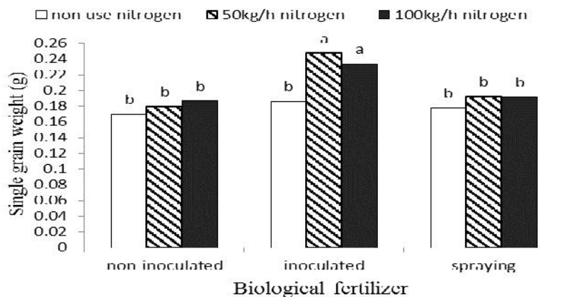
شکل ۱- اثر متقابل کود زیستی و کود اوره بر وزن تک دانه
