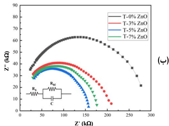
شکل ۲ طیف فوتولومینسانس (PL) (الف) و طیف رهنبدی الکترووشیمیایی (EIS) (ب) نمونه‌های چندسازه‌ای
