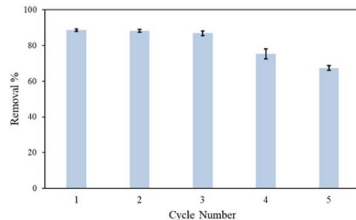
شکل ۸ تغییر میانگین درصد حذف قرمز کنگو با CQDs-pZnO بازپایی شده همراه با انحراف استاندارد برای ۳ بار تکرار در هر چرخه
