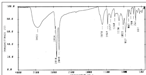
شکل ۲ طیف IR نمونه \text{MoS}_2 پوشش دار شده با PyDDP
