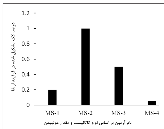
شکل ۵ مقایسه کک تشکیل شده در فرایند ارتقای کیفیت نفت فوق سنگین با درصدهای متفاوت کاتالیست
