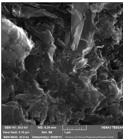
شکل ۳ تصویر SEM الکتروود بر پایه گرافن تهیه شده به روش کاهش شیمیایی و غوطه‌ورسازی
