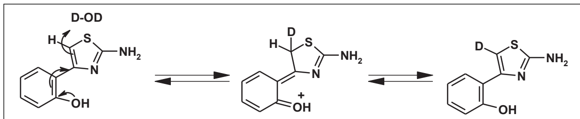
شکل ۹ چگونگی تبادل دیوتریم در ۲ - آمینوتیازول
