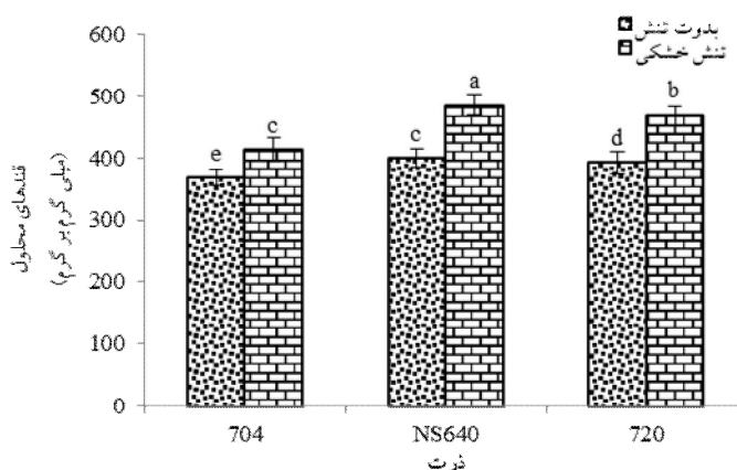
شکل ۵: تاثیر تنش خشکی و هیبریدها بر قندهای محلول ذرت طی دو سال زراعی (ستون‌های دارای حرف مشترک بر اساس آزمون مقایسه میانگین‌ها فاقد اختلاف آماری معنی دار می‌باشند)
