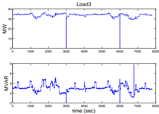
شکل ۵: پروفیل بار اکتیو و راکتیو Load3
