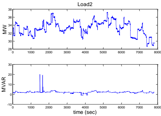
شکل ۴: پروفیل بار اکتیو و راکتیو Load2
