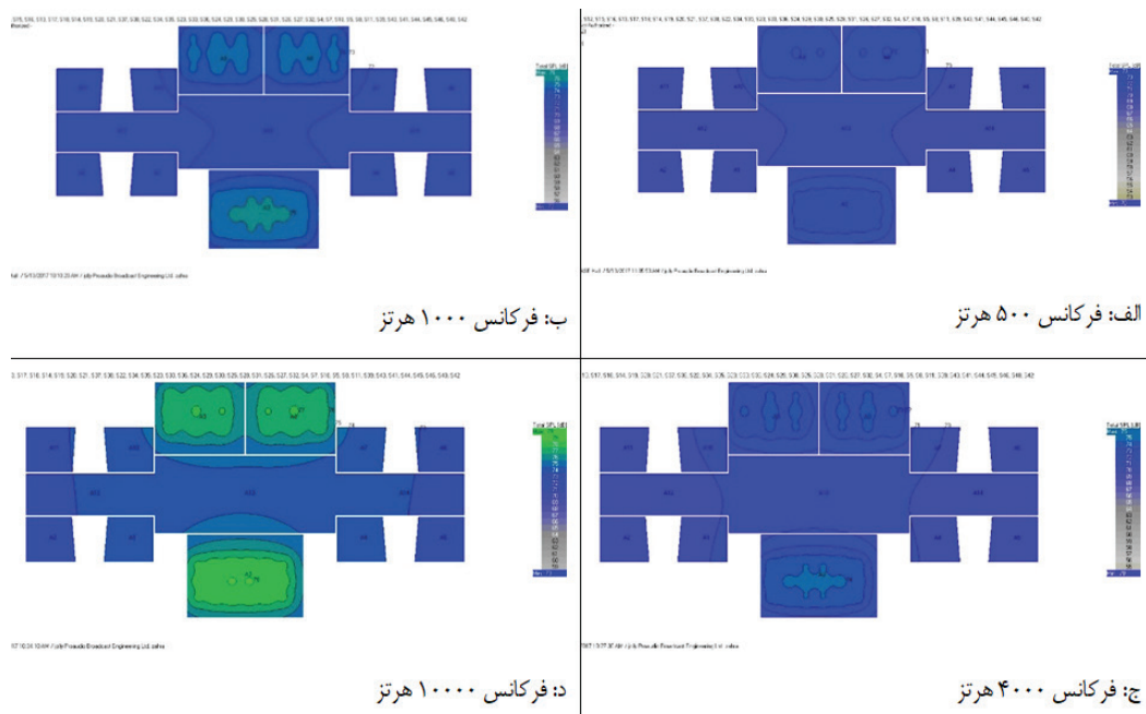
شکل ۲. وضعیت موجود تراز شدت صوت در فرکانس‌های مورد مطالعه.
