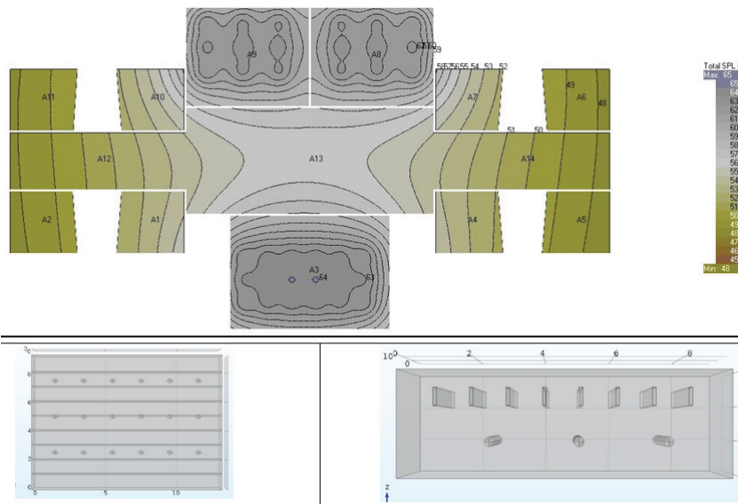
شکل ۷. وضعیت بهینه جذب‌کننده از نظر ارتفاعی
