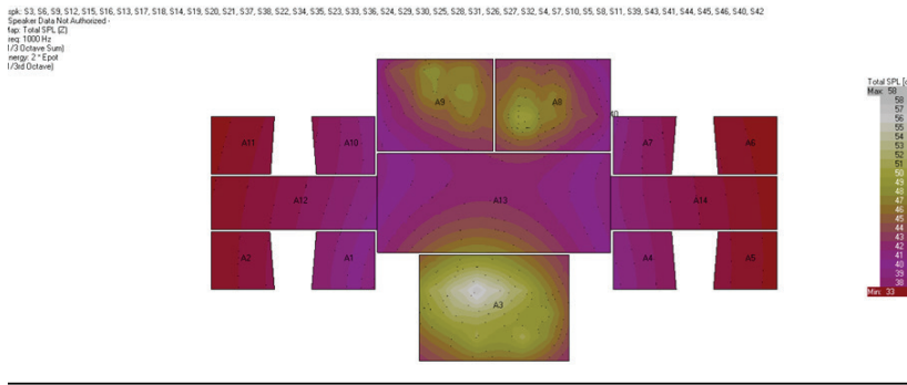
شکل ۸. جابجایی جزئی افقی در صفحات جذب کننده و تغییرات تراز شدت صوت
