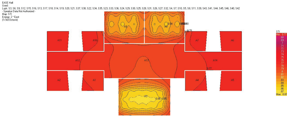
شکل ۳ ضریب انتشار صوتی در وضعیت موجود
