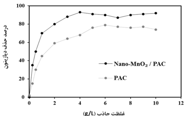
شکل (۴): ارزیابی راندمان حذف دیازینون با جاذب‌های کربن فعال کاج (PAC) و نانوکامپوزیت (Nano-MnO 2 /PAC). شرایط آزمایش: غلظت اولیه دیازینون ۲۰ mg/L، غلظت جاذب (۱۰-۲۵ g/L)، دمای محلول ۲۵ درجه سانتی‌گراد و pH=7
