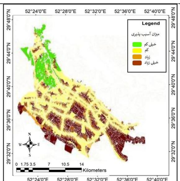
میزان آسیب پذیری شهر شیراز، بر اساس فرایندهای تکتونیکی با روش Fuzzy ANP
