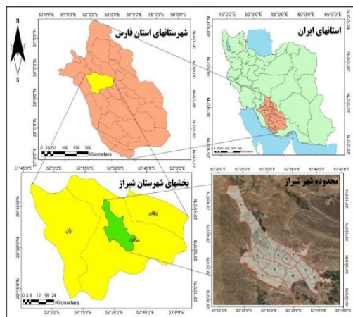
شکل ۱: موقعیت جغرافیایی و سیاسی شهر شیراز در کشور منبع: نگارنده
