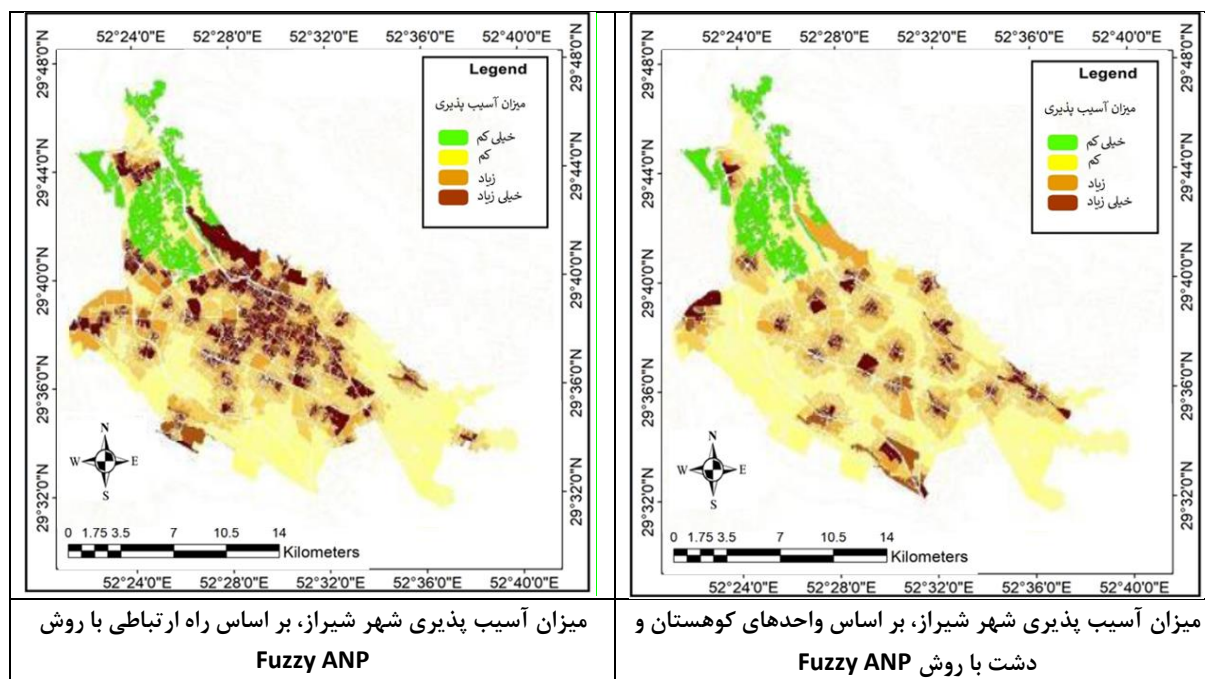
شکل ۲: میزان آسیب پذیری شیراز آسیب پذیری شهر شیراز بر اساس عوارض ژئومورفولوژیک منبع: نگارنده
