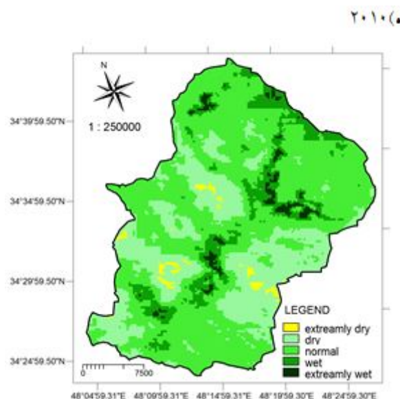
شکل (۶): نقشه پهنه بندی شاخص خشکسالی سلامت گیاهی
