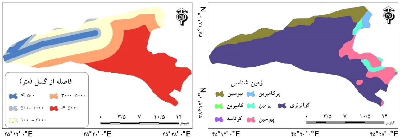
شکل ۴. نقشه زمین شناسی و فاصله از گسل
