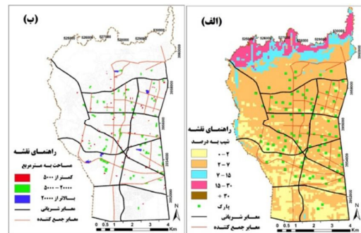
شکل (۴): شیب محدوده مورد مطالعه و موقعیت و مساحت پارک‌های محله‌ای در آن
