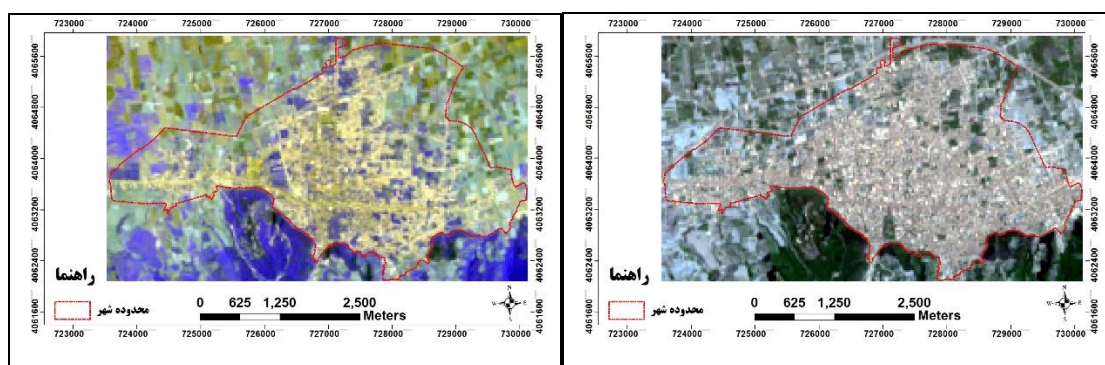
شکل (۳): تصویر OLI ماهواره لندست ۸ (ژوئن ۲۰۲۰).
