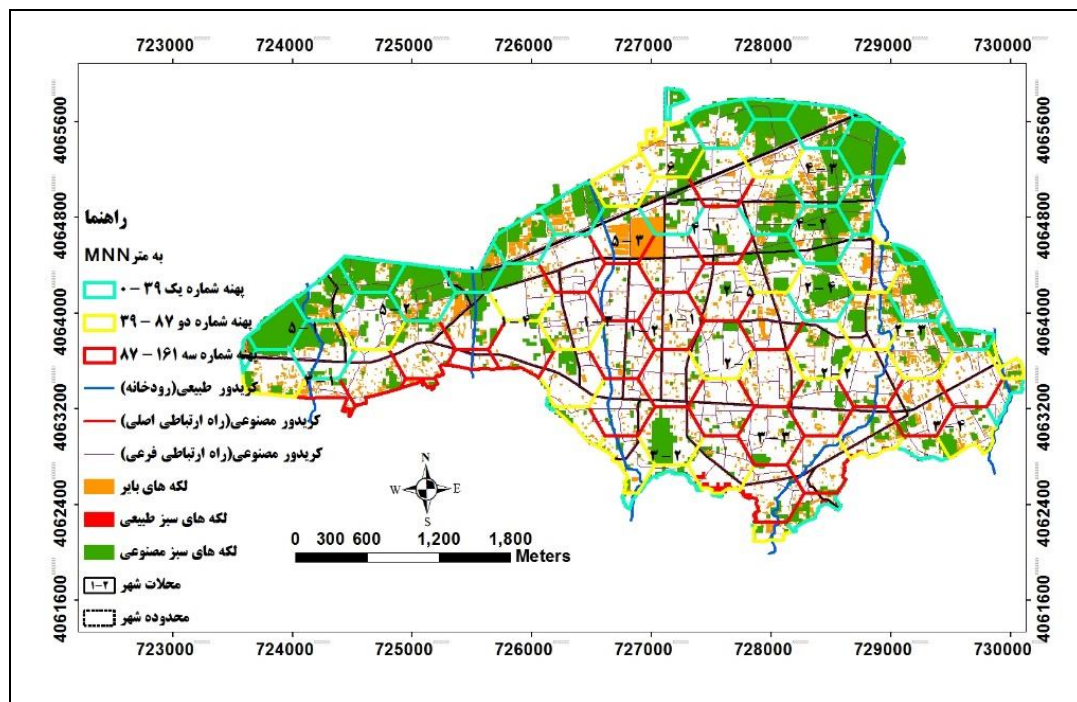
شکل (۱۰): رویهم گذاری لکه‌ها و کریدورهای طبیعی و مصنوع موجود بر روی پهنه‌های حاصل از متریک MNN
