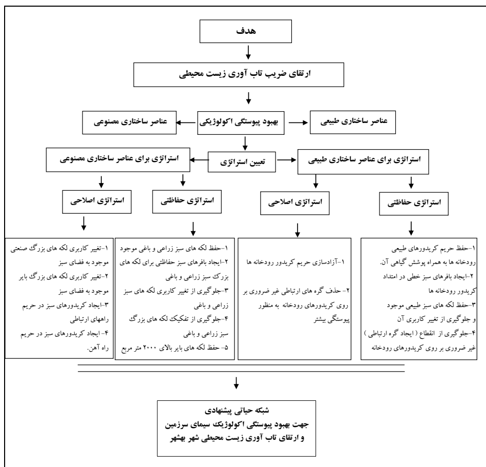
شکل (۱۱): نمودار الگوی پیشنهادی تحقیق جهت بهبود پیوستگی اکولوژیک سیمای سرزمین و ارتقای تاب‌آوری زیست محیطی شهر به‌شهر (ماخذ: نگارنده، ۱۴۰۰).
