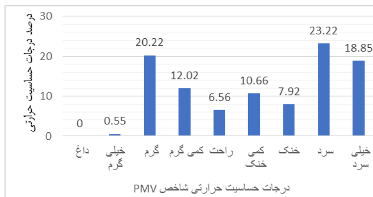
شکل (۳): درصد طبقات حساسیت حرارتی در یک سال در شهر یاسوج بر اساس شاخص PMV
