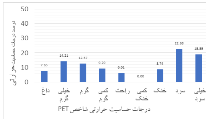
شکل (۲): درصد طبقات حساسیت حرارتی در یک سال در شهر یاسوج بر اساس شاخص PET
