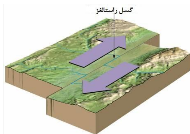
شکل ۳. گسل راستالغز
