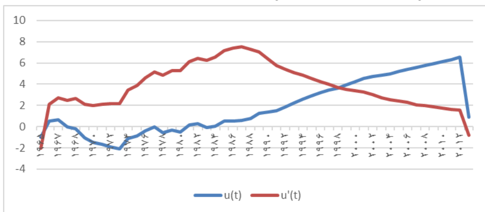
شکل شماره ۳- مقادیر دمای حداقل سالانه ایستگاه اهواز Research findings Source:
