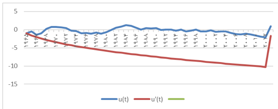
شکل شماره ۹- مقادیر u و u' سالانه رطوبت نسبی ایستگاه اهواز Research findings Source:
