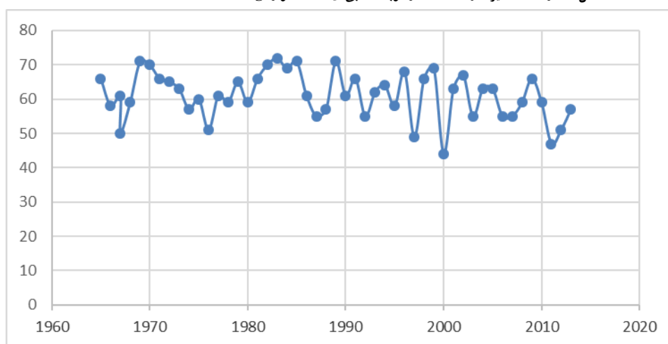
شکل شماره ۱۰- مقادیر سالانه رطوبت نسبی ایستگاه اهواز Research findings Source:
