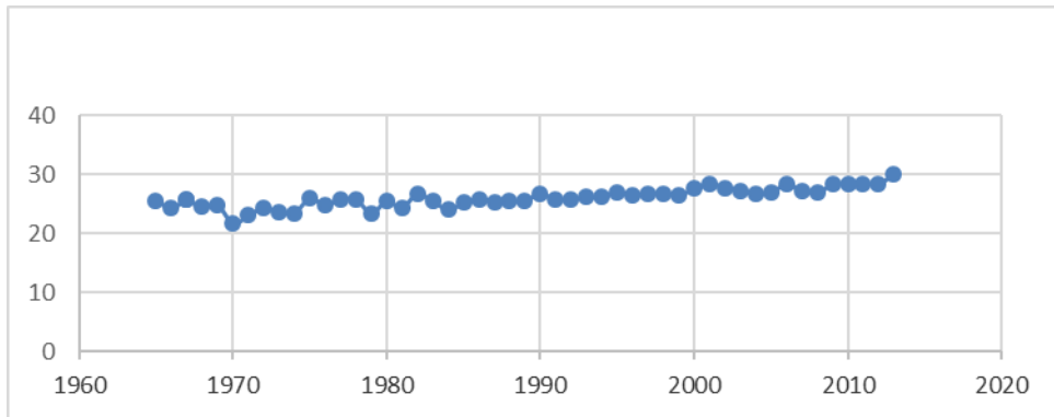
شکل شماره ۲- مقادیر u و u' دمای حداقل سالانه ایستگاه اهواز Research findings Source:
