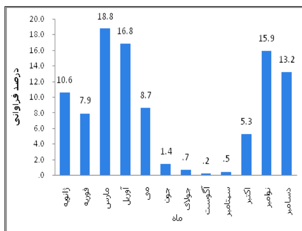
شکل (۲): درصد فراوانی تیپ بارش‌مند در ماههای مختلف سال در مراغه
