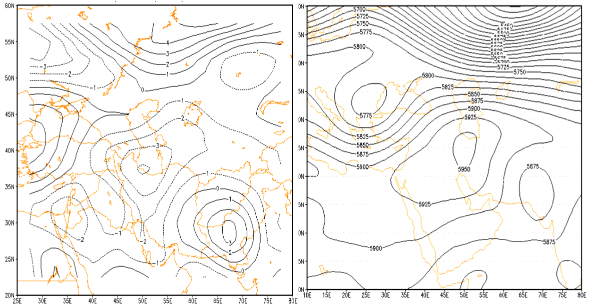
شکل (۱۸): الگوی گردشی فشار و تاوایی تراز میانی (۵۰۰ هکتوپاسکال) تیپ گرم و خشک
