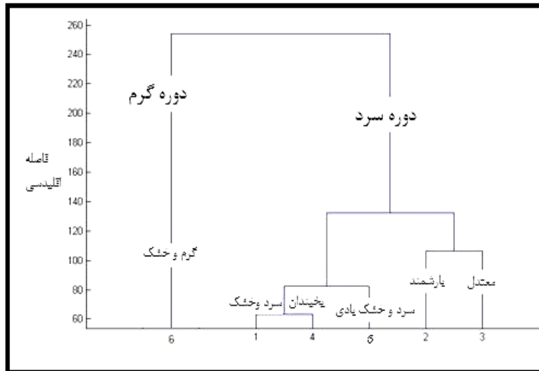
شکل (۱): دارنمای شش تیپ اقلیمی ایستگاه مراغه
