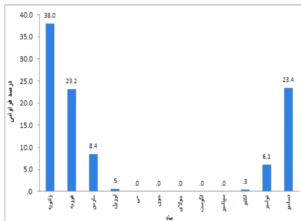
شکل (۱۰): درصد فرآوانی تیپ یخبندان در ماههای مختلف سال در مراغه
