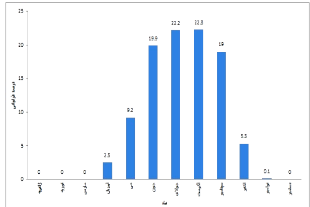
شکل (۱۳): فرآوانی تیپ گرم و خشک و تغییرات سالانه آن در مراغه
