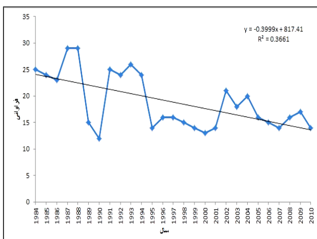
شکل (۳): فراوانی تیپ بارش‌مند و تغییرات سالانه آن در طول دوره آماری در مراغه
