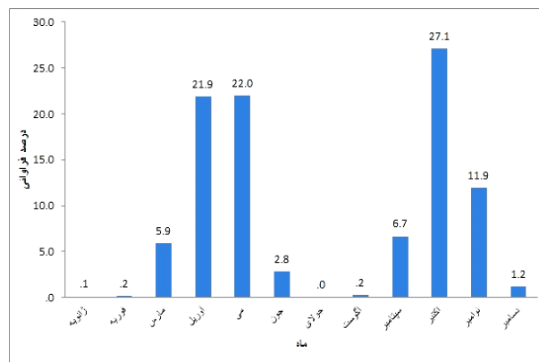
شکل (۸): درصد فرآوانی تیپ معتدل در ماههای مختلف سال در مراغه
