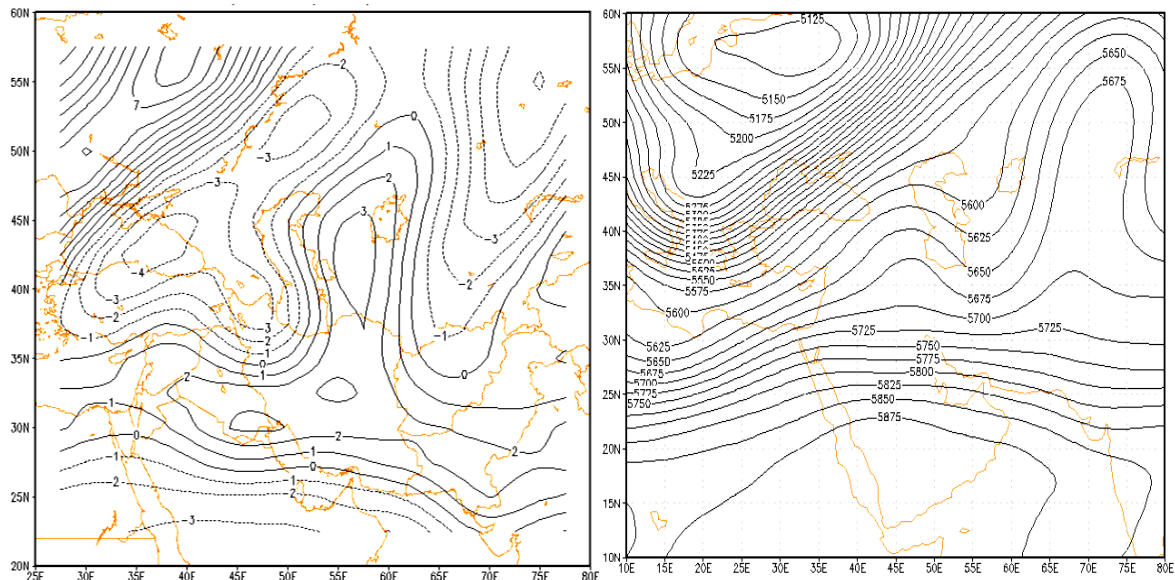
شکل (۱۶): الگوی گردشی فشار و تاوایی تراز میانی (۵۰۰ هکتوپاسکال) تیپ سرد و خشک بادی
