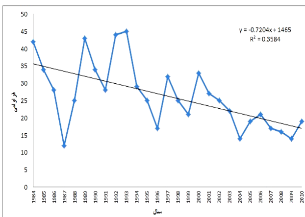
شکل (۱۱): فرآوانی تیپ یخبندان و تغییرات سالانه آن در مراغه
