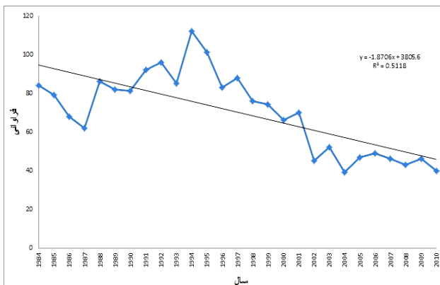
شکل (۹): فرآوانی تیپ معتدل و تغییرات سالانه آن در مراغه
