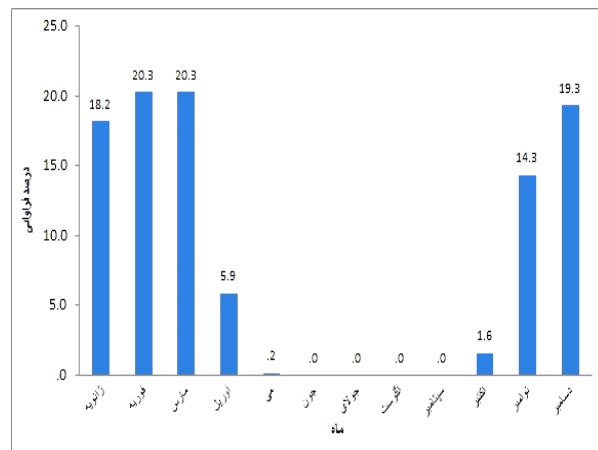
شکل (۴): درصد فراوانی تیپ سرد و خشک در ماههای مختلف سال در مراغه
