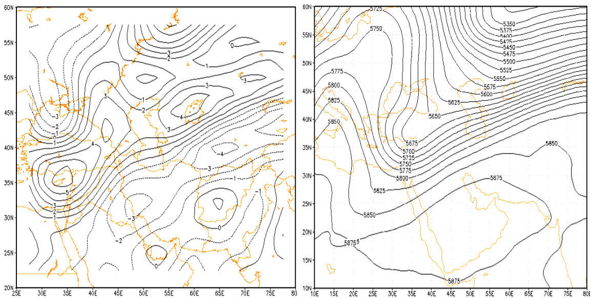
شکل (۱۴): الگوی گردشی فشار و تاوایی تراز میانی (۵۰۰ هکتوپاسکال) روز نماینده تیپ بارشی
