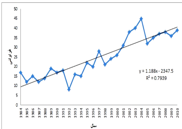
شکل (۷): فرآوانی تیپ سرد و خشک بادی و تغییرات سالانه آن در مراغه
