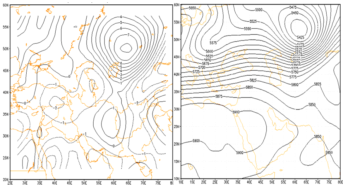
شکل (۱۷): الگوی گردشی فشار و تاوایی تراز میانی (۵۰۰ هکتوپاسکال) تیپ معتدل
