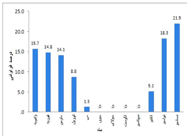
شکل (۶): درصد فرآوانی تیپ سرد و خشک بادی در ماههای مختلف سال در مراغه
