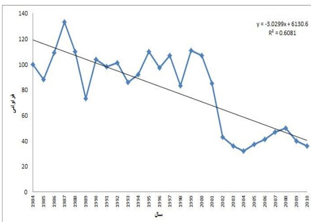
شکل (۵): فراوانی تیپ سرد و خشک و تغییرات سالانه آن در مراغه
