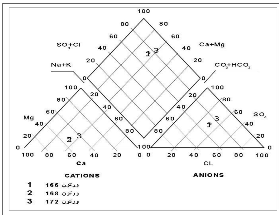
شکل ۵- آب های منطقه ورتون در دیاگرام یابیر
