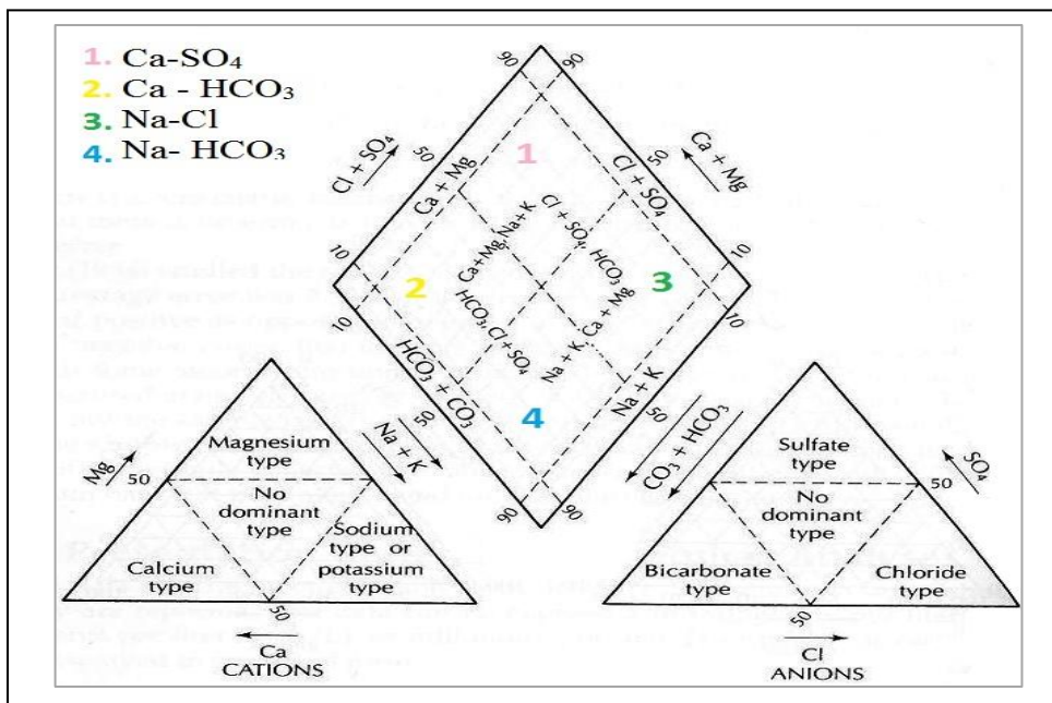
شکل ۴- دیاگرام یابیر منشاء آب ها و موقعیت چشمه ورتون
