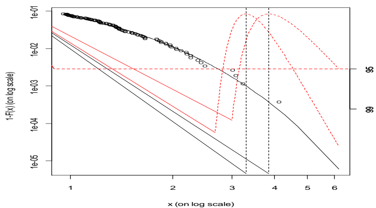
شکل ۱۹- دم تخمین زده توسط مدل GPD با آستانه ۰,۹۵ و نمایش شماتیک VAR (از سمت چپ منحنی اول) و ES (از سمت چپ منحنی دوم)
