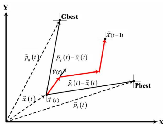
شکل (۳): نحوه‌ی عملکرد الگوریتم بهینه‌سازی ازدحام ذرات
