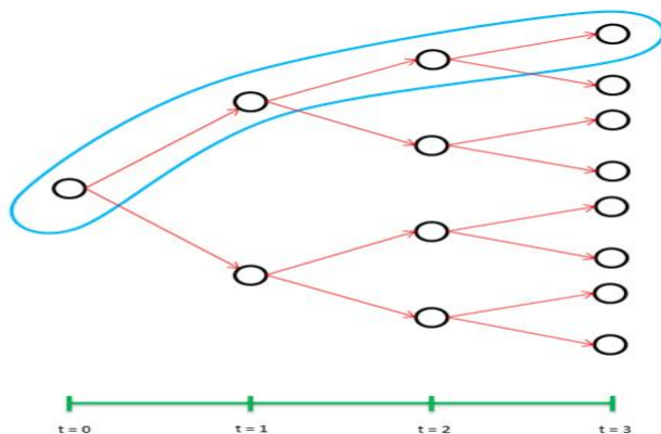
شکل (۱): درخت سناریو با ۳ مرحله و ۸ سناریو
