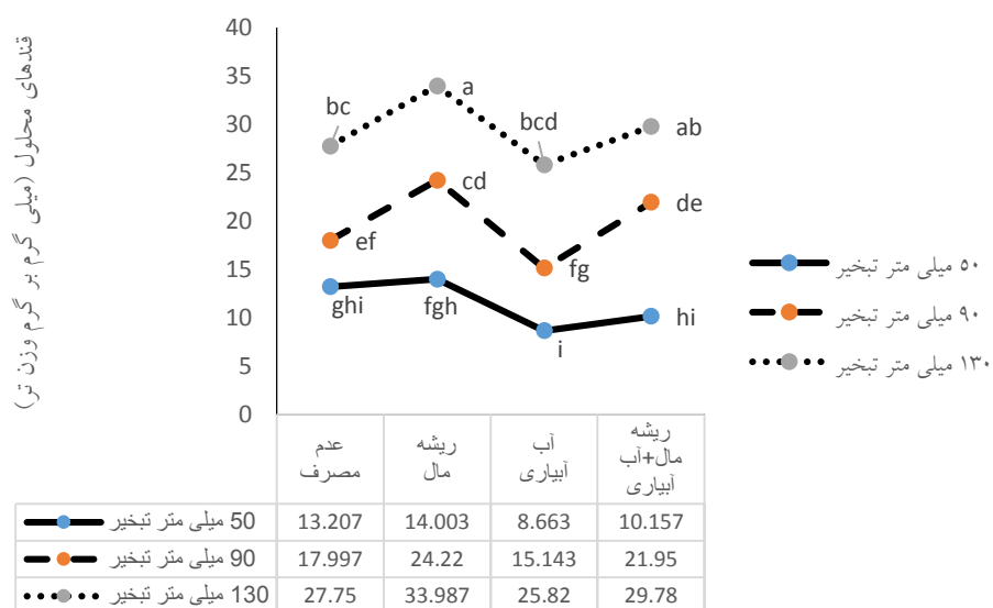
شکل ۲- اثر متقابل سطوح آبیاری و روش‌های کاربرد باکتری‌های محرک رشد بر میزان قندهای محلول در برگ بومادران
