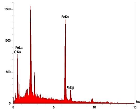
شکل ۵: تصویر میکروسکوپ الکترونی ریشی (SEM) نانو ذرات اکسید آهن سنتز شده با استفاده از عصاره آبی گیاه خرفه و طیف پراش اشعه ایکس (EDX) مربوط به آن.
