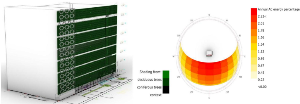
شکل ۱۳. میزان انرژی جریان متناوب سالانه برحسب مسیر تابش خورشید
