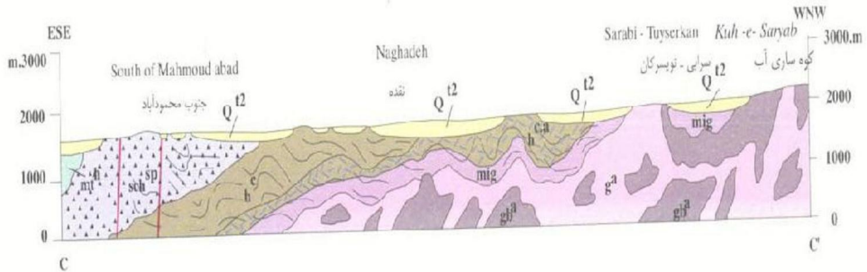
شکل ۲- چینه‌شناسی جنوب شرقی ورقه توپسرکان (منبع: طرح جامع شهر توپسرکان)
