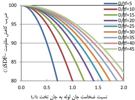
شکل ۶: مقدار SDF برای مقادیر مختلف D/t_f و t_w/t_f
