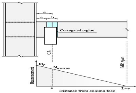
شکل ۱۳: توزیع لنگر در اتصال
