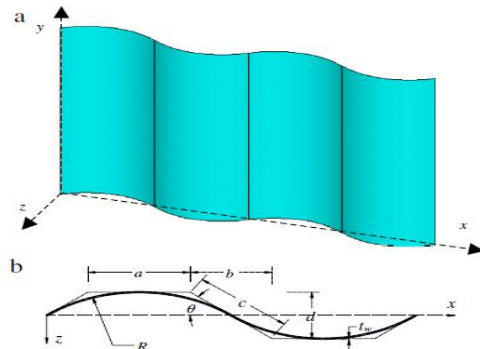
شکل ۱۲: مشخصات هندسی ورقهای موج‌دار کمناشی
