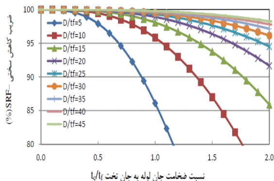
شکل ۴: مقدار SRF برای مقادیر مختلف t_c/t_f و D/t_f
