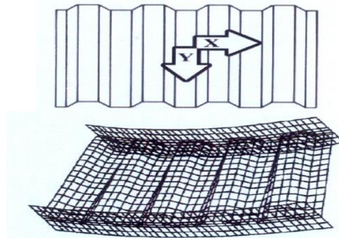
شکل ۱: ورق موج دار
