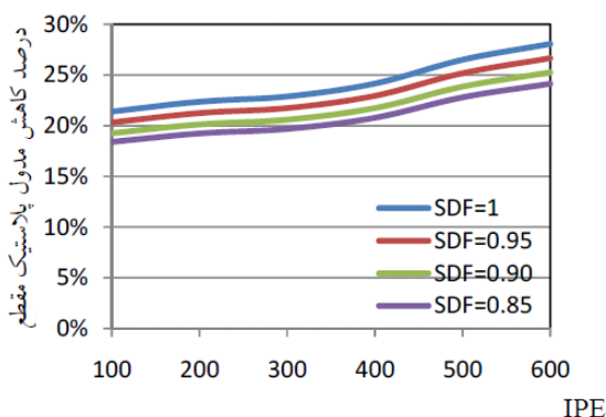
شکل ۸: درصد کاهش ممان اینرسی و مدول مقطع پلاستیک تیر در اتصال TW-RBS
