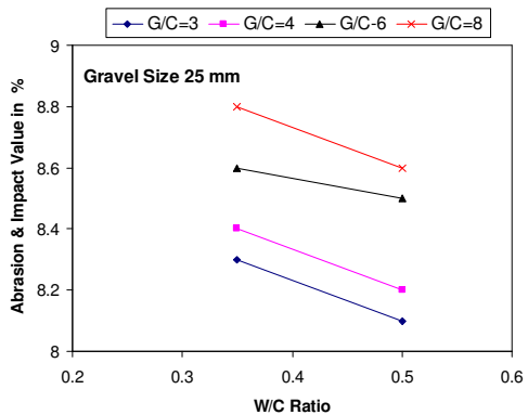
شکل ۷. رابطه نسبت آب به سیمان و قطر دانه درشت در مقاومت سایشی-ضربه ای بتون فاقد ریزدانه
