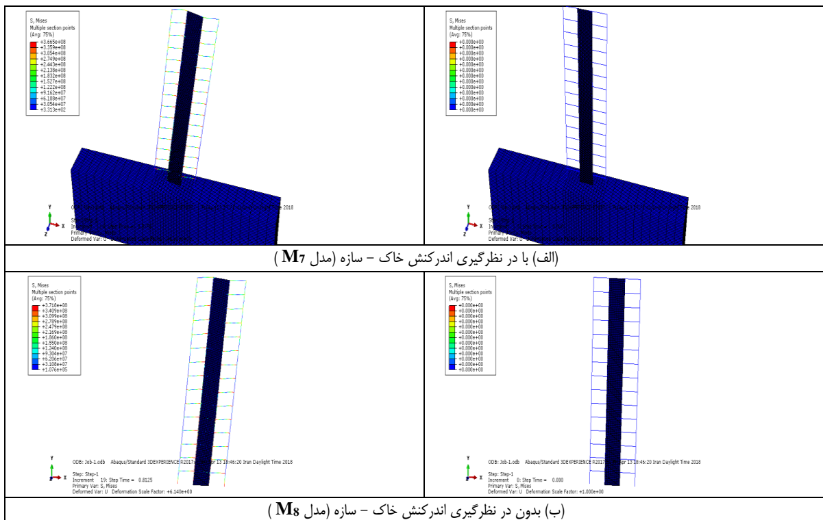
شکل ۶- نمونه مدل سازی شده و خطوط همتراز تنش تسلیم در سازه ۱۵ طبقه با دیوار برشی بتنی در نرم افزار ABAQUS جدول ۴- نتایج تحلیل های پاسخ سازه برای مدل های مختلف در سازه های ۱۰ و ۱۵ طبقه
