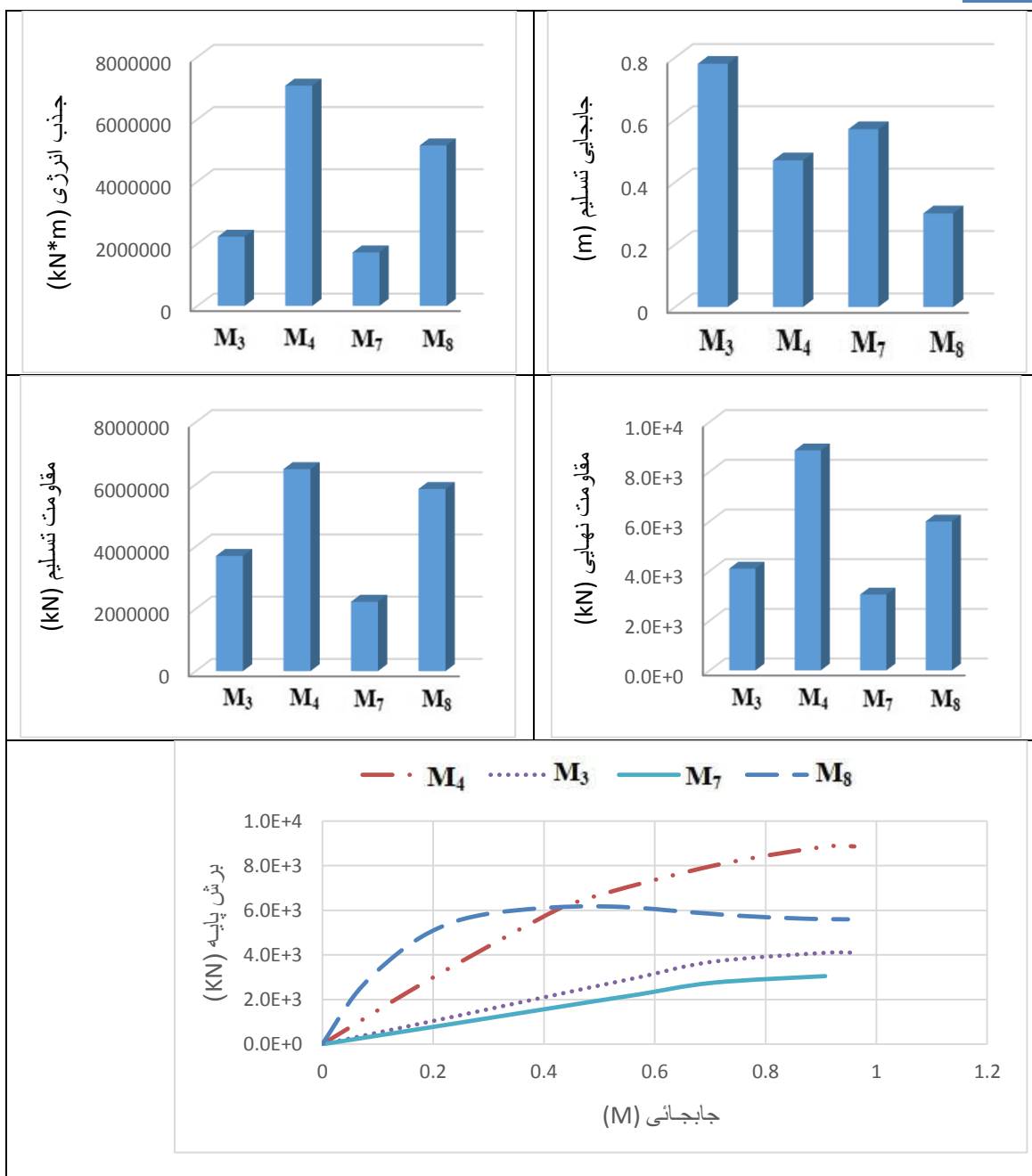
شکل ۸- مقایسه نتایج مربوط به پاسخ رفتار سازه‌های ۱۵ طبقه دارای سیستم‌های دیوار برشی‌های فولادی و بتنی
