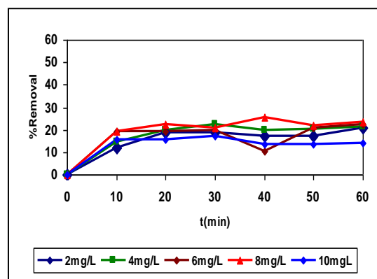
نمودار ۲- تاثیر غلظت اولیه 4C2NP بر میزان حذف آن در فرآیند
