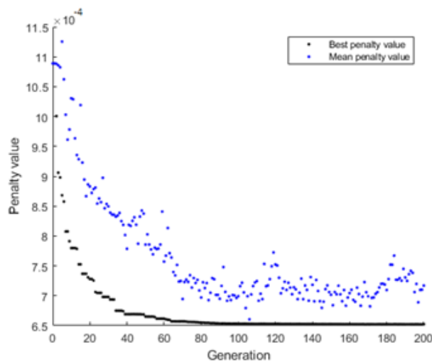
شکل (۲): تابع هزینه در الگوریتم ژنتیک برای انتخاب الکترود بهینه Figure (2): Cost function in the genetic algorithm for optimal electrode selection
