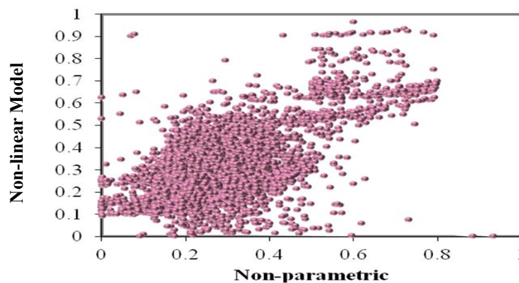
شکل ۲. نمودار پراکنندگی داده‌های مدل غیرخطی و ناپارامتریک
