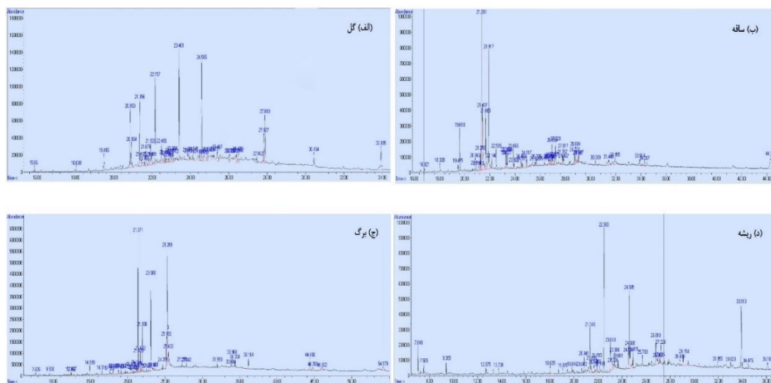
شکل ۱: کروماتوگرام‌های GC-MS فرکشن‌های کلروفومی: (الف) گل، (ب) ساقه، (ج) برگ و (د) ریشه
