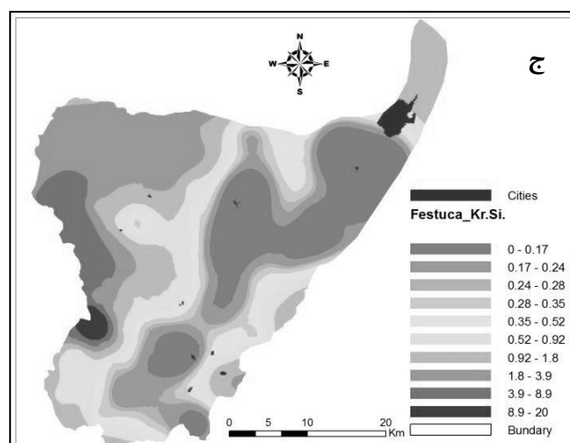
شکل ۳- نقشه‌های میان‌بازی تاج پوشش گونه F. ovina در منطقه مورد مطالعه (الف)، روش معکوس وزنی فاصله؛ (ب)، روش کریجینگ معمولی؛ (ج)، روش کریجینگ ساده
