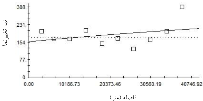
شکل ۲- تغییرنمای حاصل از تاج پوشش گونه F. ovina
