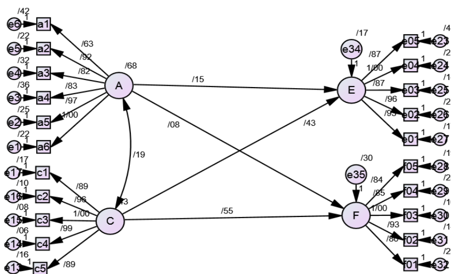
نمودار شماره (۲): مدل معادله ساختاری
