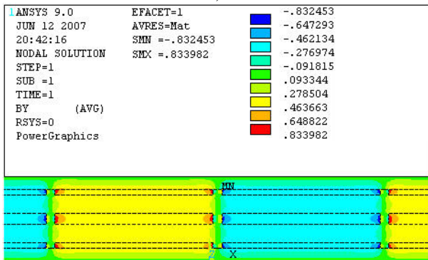
Fig. 8 Result of FEM
