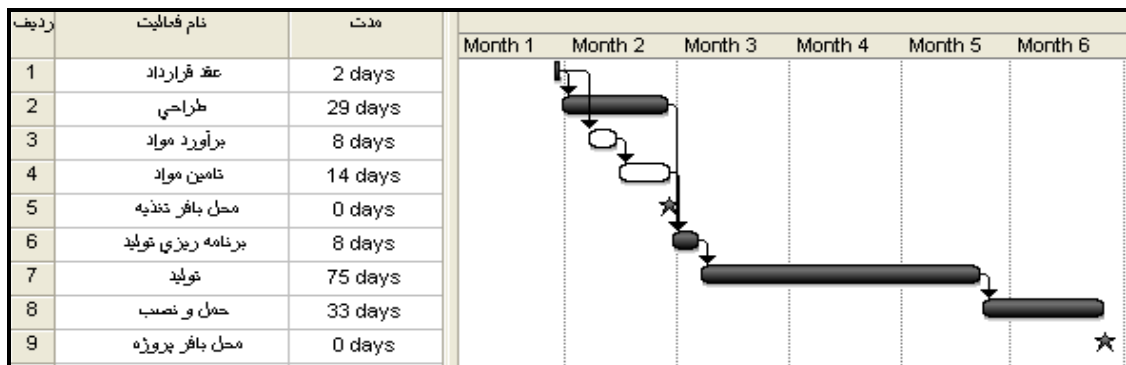
شکل شماره (۴): زنجیره بحرانی و محل قرار گرفتن بافرها
