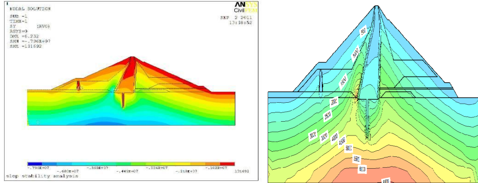
شکل 2: توزیع تنش قائم در ansys و geo studio
