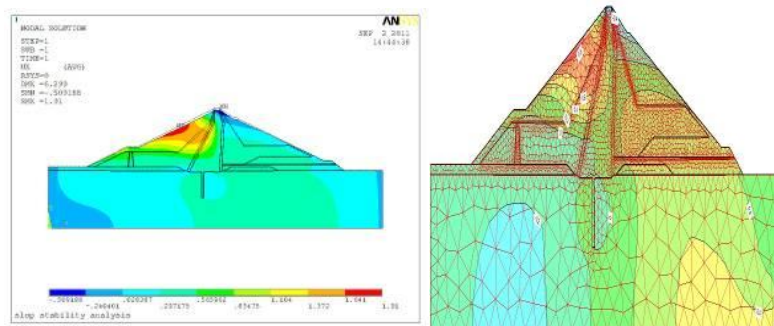
شکل 6: جابجایی در راستای افقی در geo studio و Ansys
