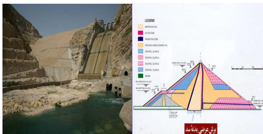
شکل 1: سد مارون و مقطع تیپ سد مارون
