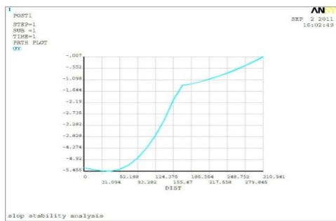
شکل 8: جابجایی قائم در ansys و geo studio
