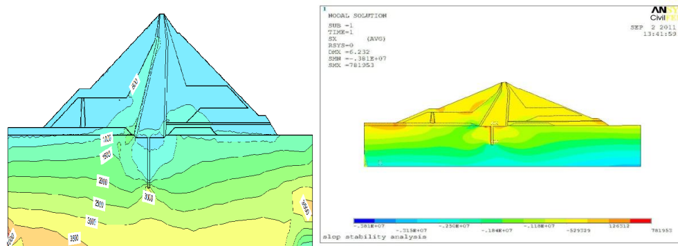
شکل 3: توزیع تنش افقی در ansys و geo studio
