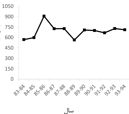
شکل ۳: تغییرات EC در ایستگاه تنگ پنج سزار
