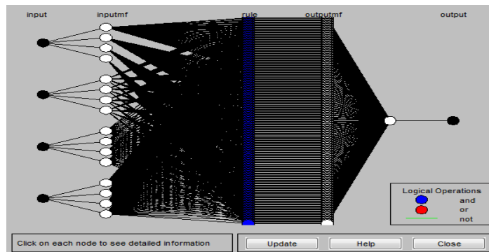
شکل ۵: ساختار مدل شبکه عصبی تطبیقی تهیه شده
