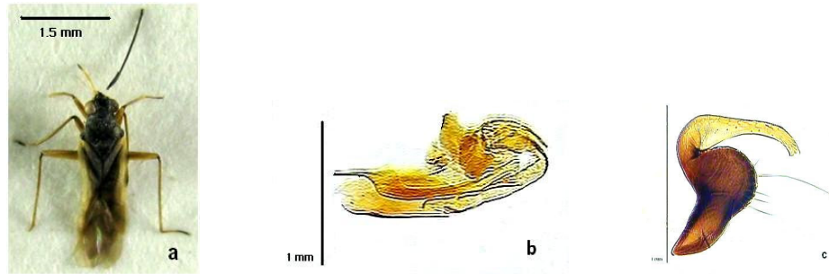
شکل ۱- الف- حشره کامل نر Cyrtorhinus caricis ب- Aedeagus ج- پارامر چپ Fig 1- a- Cyrtorhinus caricis male b- structure of Aedeagus c-left paramer
