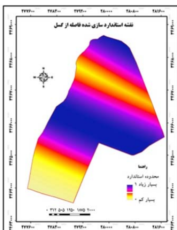
گسل
