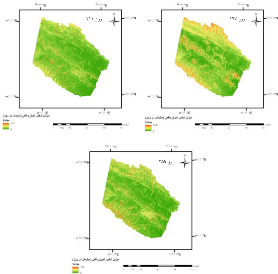
شکل ۷. مقادیر تبخیر-تعرق واقعی برحسب (mm/day) بر اساس الگوریتم مثلثی در روزهای ۱۴۷، ۲۱۱ و ۲۵۹ سال ۲۰۲۰.
