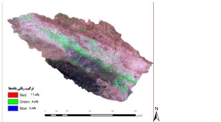
شکل ۲. کاربری اراضی منطقه مورد مطالعه بر اساس تصاویر ماهواره سنتینل ۲، ترکیب باندهای (باند های ۱۱، ۸ و ۴).
