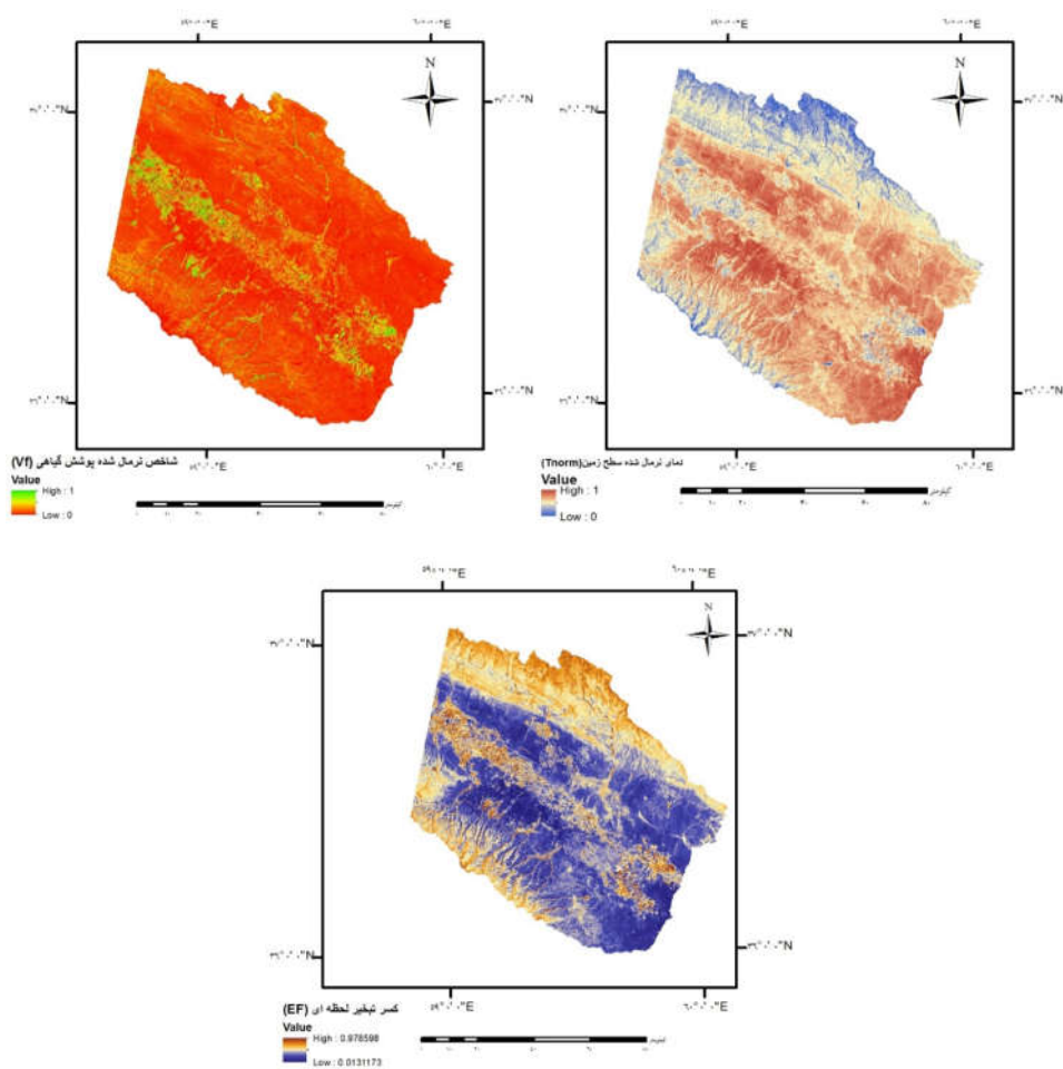
شکله. مقادیر نرمال شده پوشش گیاهی، نرمال شده دمای سطح زمین و میزان کسر تبخیر لحظه ای برای روز ۱۴۷ سال ۲۰۲۰.
