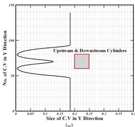
شکل (۲): توزیع اندازه حجم‌های کنترل شبکه ایجاد شده، الف) در امتداد محور X ب) در امتداد محور Y
