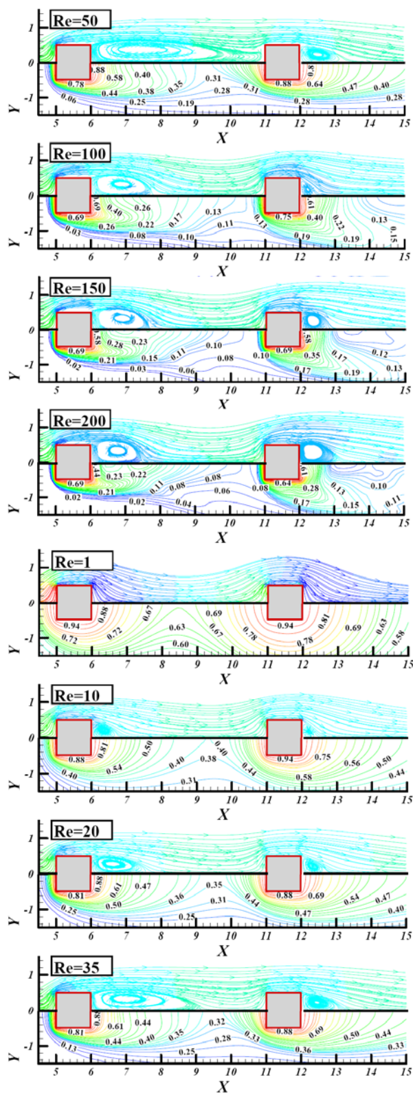
شکل (۵) خطوط جریان رنگ شده توسط فشار (نیمه بالایی تصاویر) و دما ثابت (نیمه پایینی تصاویر) نواحی اطراف سیلندرها در اعداد رینولدز مختلف در محدوده جریان دائم (تصاویر سمت چپ) و جریان غیردائم-متوسط‌گیری (تصاویر سمت راست)
