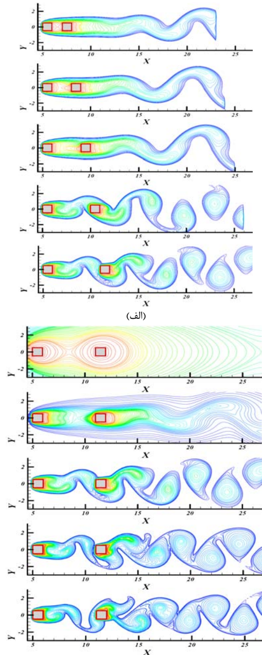
شکل (۶) الگوی دمایی لحظه‌ای نواحی اطراف سیلندرها در مقابل (الف) افزایش فاصله بین سیلندری G=1-5 برای Re=100 ، (ب) افزایش عدد رینولدز Re=1,500, 1,000, 1,500, 2,000 برای G=5
