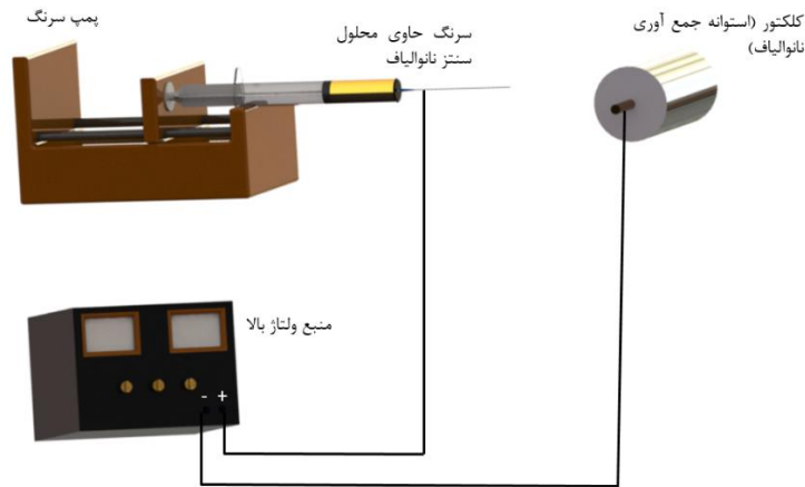
شکل ۲: شماتیک فرآیند الکتروروسی نانوالیاف و تجهیزات مورد نیاز.
