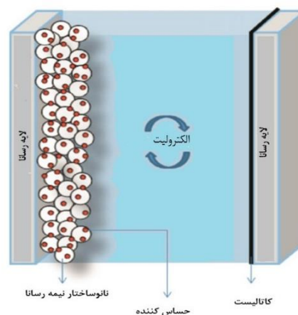
شکل ۱: ساختار و فرآیند کاری سلول خورشیدی DSSC.
