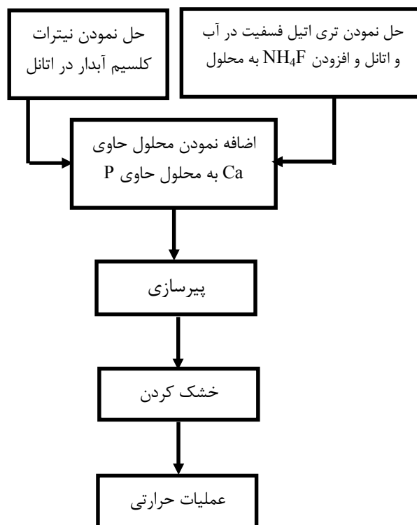
شکل ۱: دیاگرام تهیه نانوکامپوزیت فلئور- هیدروکسی آپاتیت (FHAp) به روش سل-زل.
