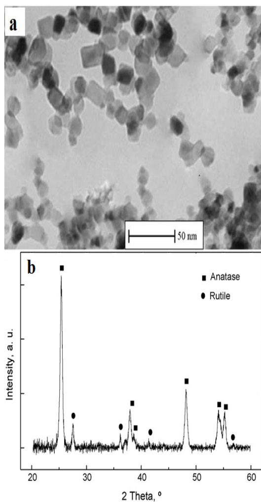
شکل ۳: TEM (a) و XRD نانوپودر \text{TiO}_2 (b).
