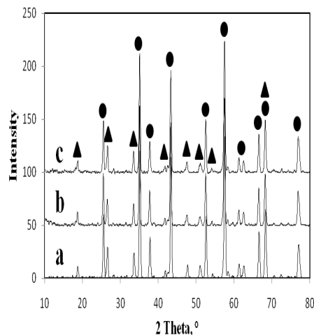
شکل ۶: الگوی پراش اشعه ایکس (XRD) نمونه‌های زینتر شده در دماهای ۱۳۰۰°C (a)، ۱۴۰۰°C (b) و ۱۵۰۰°C (c). ●: آلومینیوم تیتانات، ▲: آلفا آلومینا.
