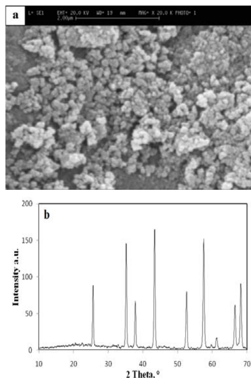
شکل ۲: SEM (a) و XRD نانو پودر \text{Al}_2\text{O}_3 (b).
