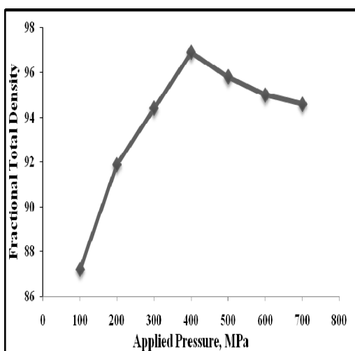
شکل ۵: دانسیته نمونه‌های زینتر شده در دمای 1500^{\circ}\text{C} در فشار پرس‌های مختلف.
